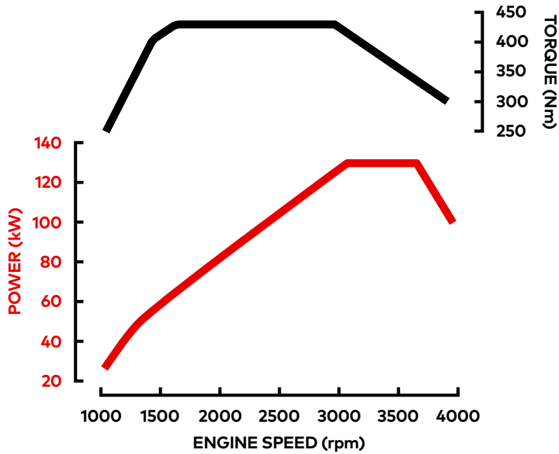
Fuso 4P-10 T6
