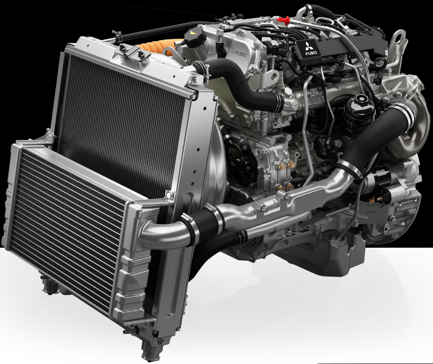
Fuso 4P-10 T6
